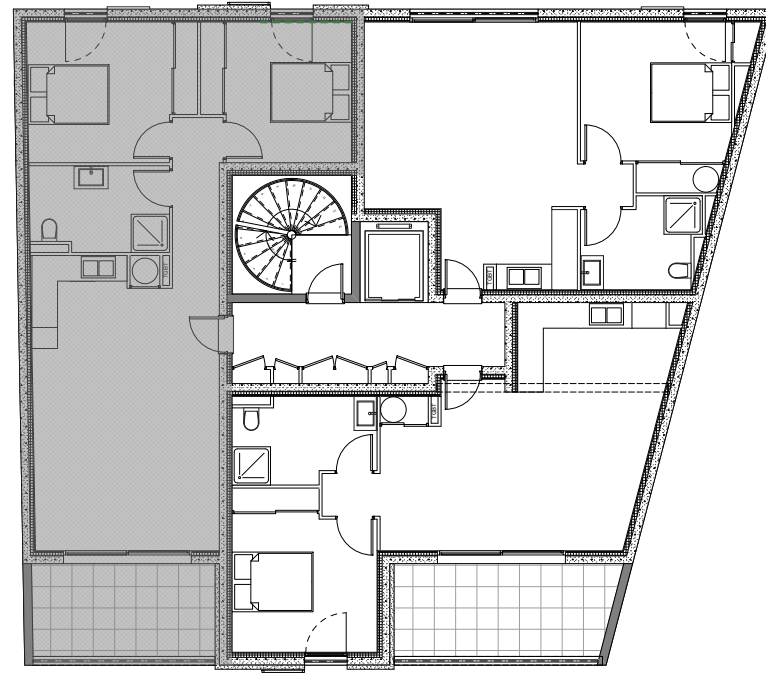
Plan d'étage courant R+3
